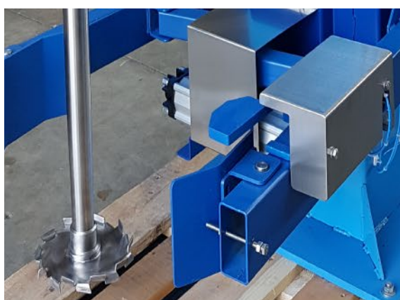
Dettaglio propeller con dispositivo centraggio e ritegno fusti
